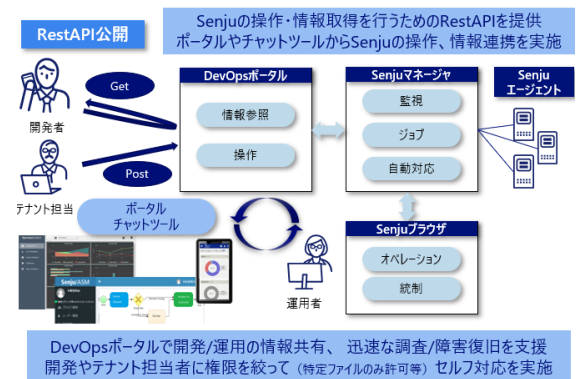
※RestAPIによる外部連携イメージ
