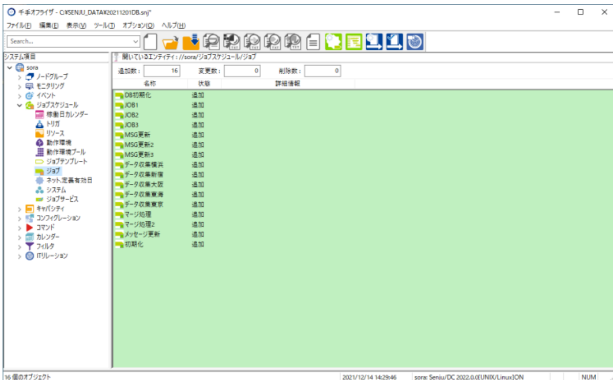
図 4.39 差分表示モード
