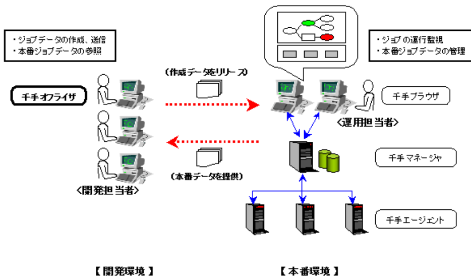
図 2.1 千手オフライザを用いたシステム構成例
