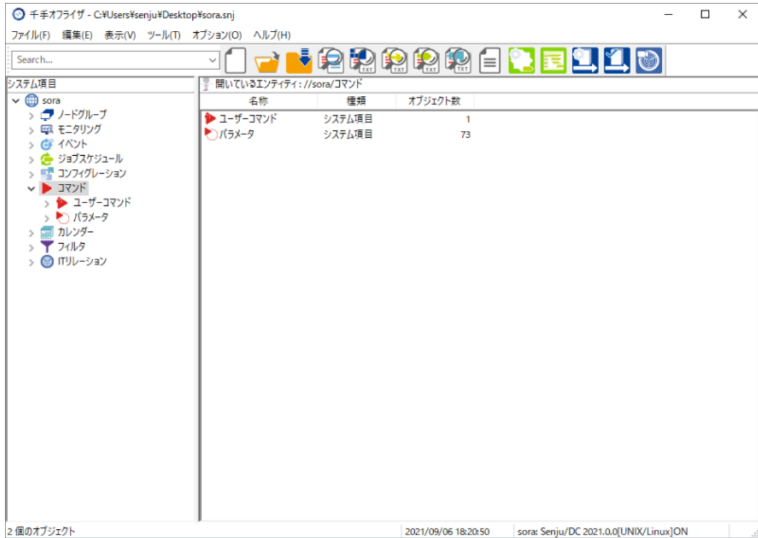
図 3.24 コマンドのエンティティ
