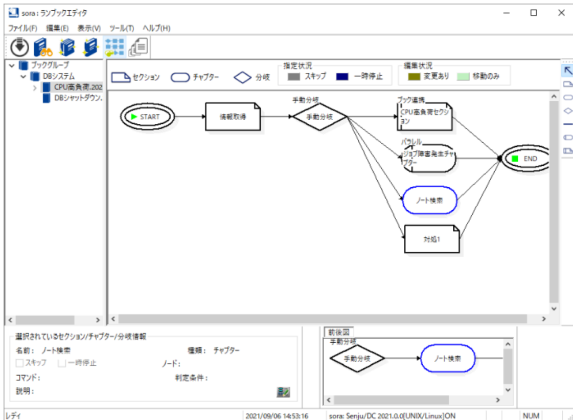
図 4.10 ランブックエディタ
