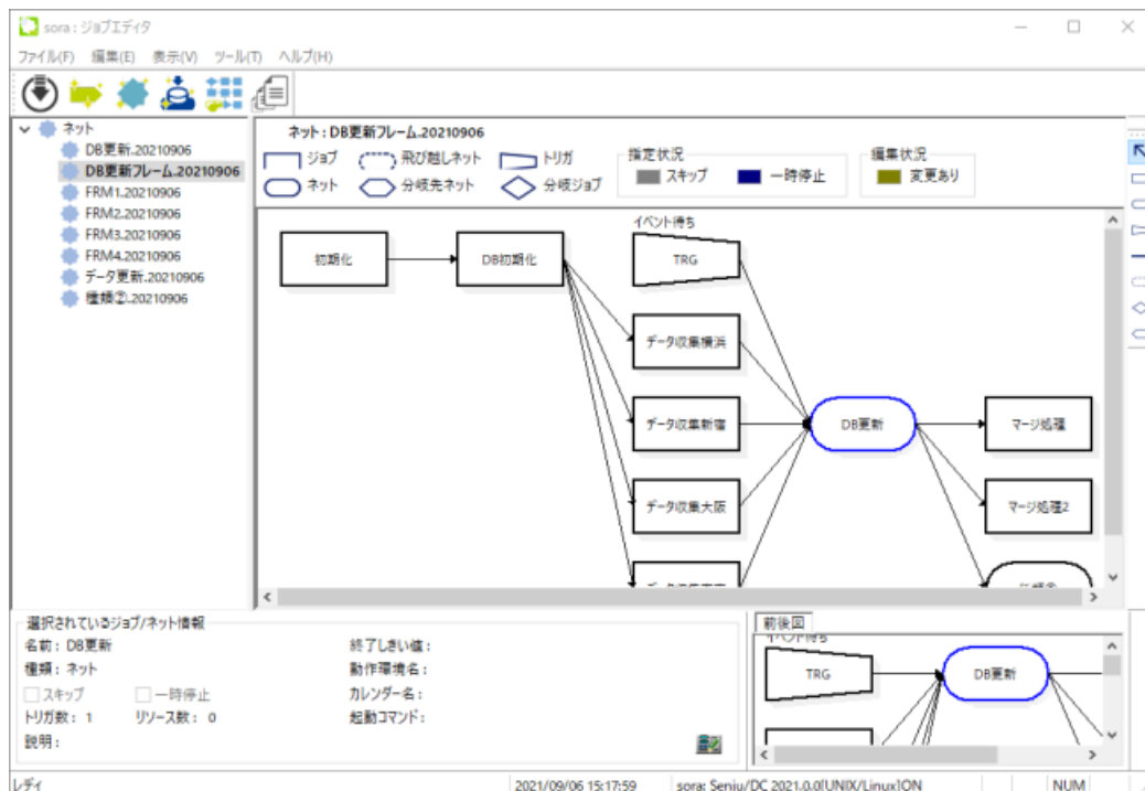
図 4.11 ジョブエディタ
