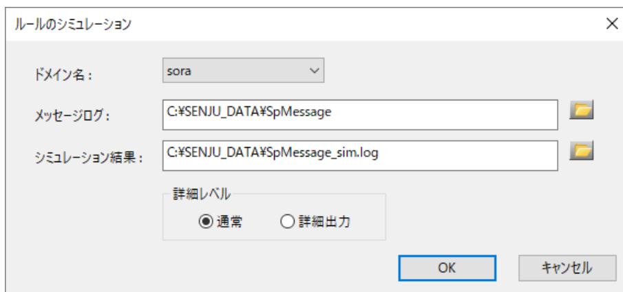
図 4.41 ルールのシミュレーションダイアログ
