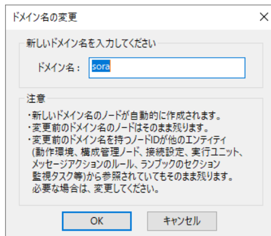
図 4.25 ドメイン名の変更ダイアログ
