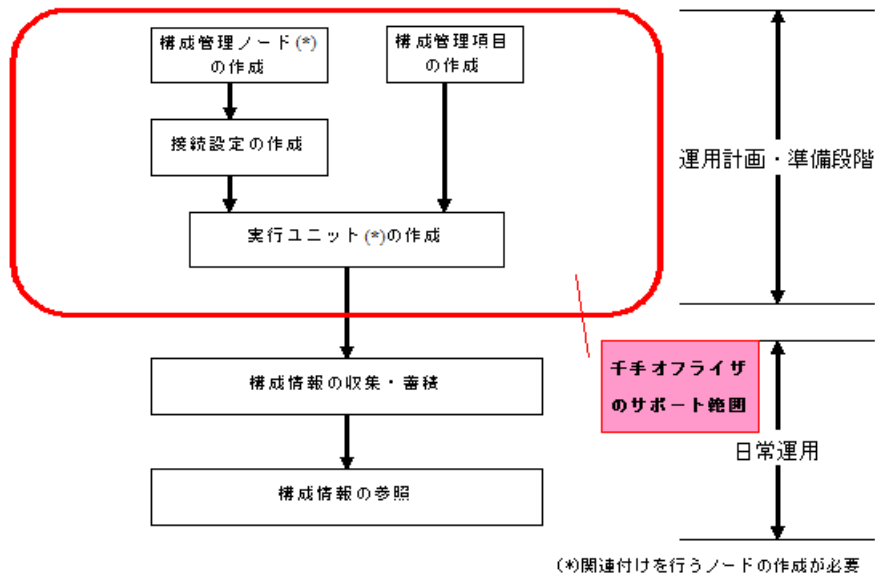
図 4.4 コンフィグレーションの流れ
